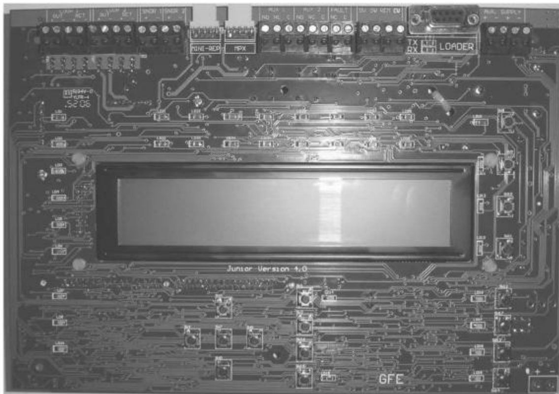
VISTA FRONTALE
