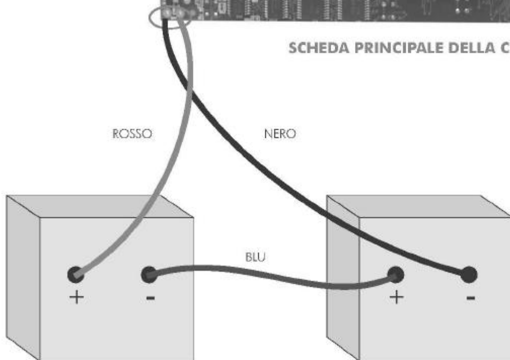
BATTERIE DELLA CENTRALE
