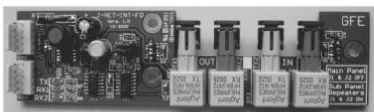
SCHEDA INTERFACCIA PER FIBRE OTTICHE
