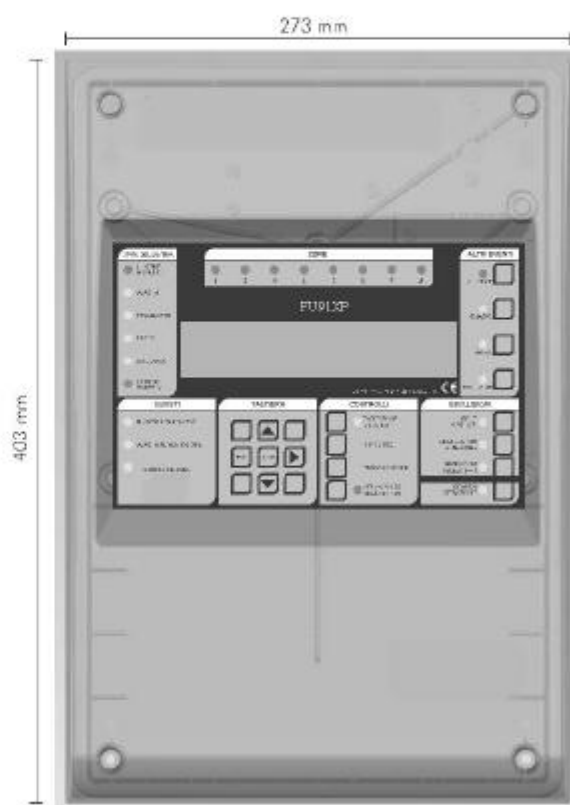
VISTA FRONTALE
